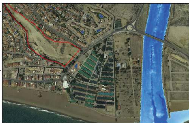
CALADO. T=10 AÑOS. SNCZI
