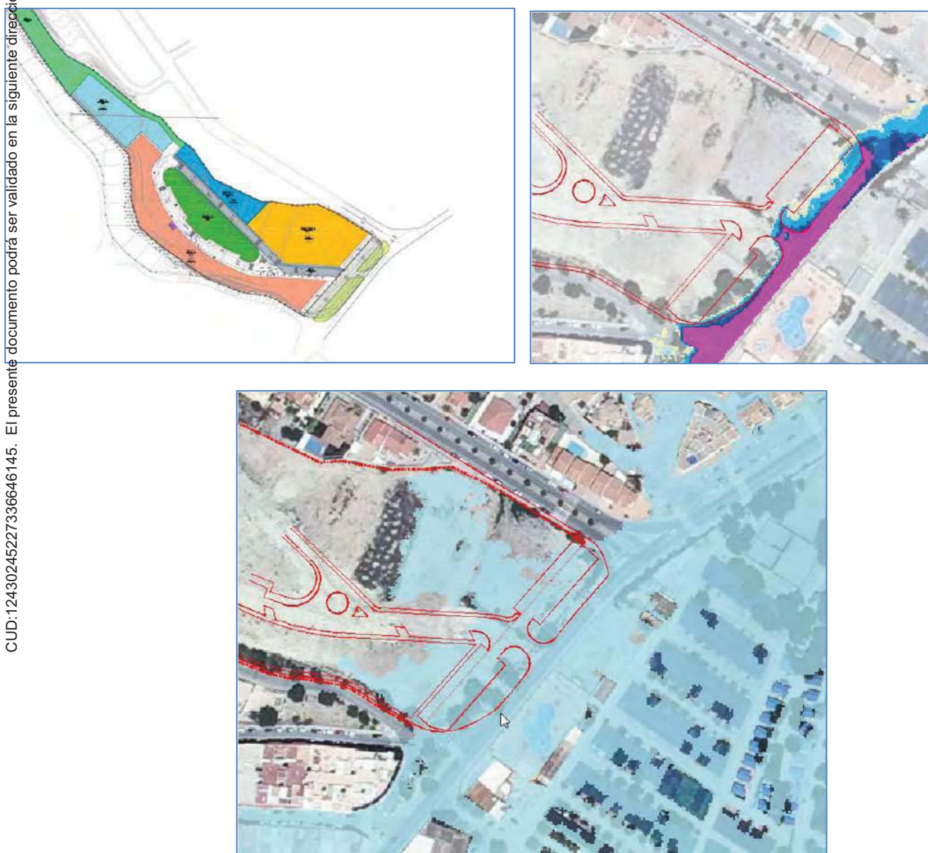
Vista de la propuesta de ordenación, la lámina de inundación en la situación futura y la lámina de inundación en la situación actual, respectivamente
