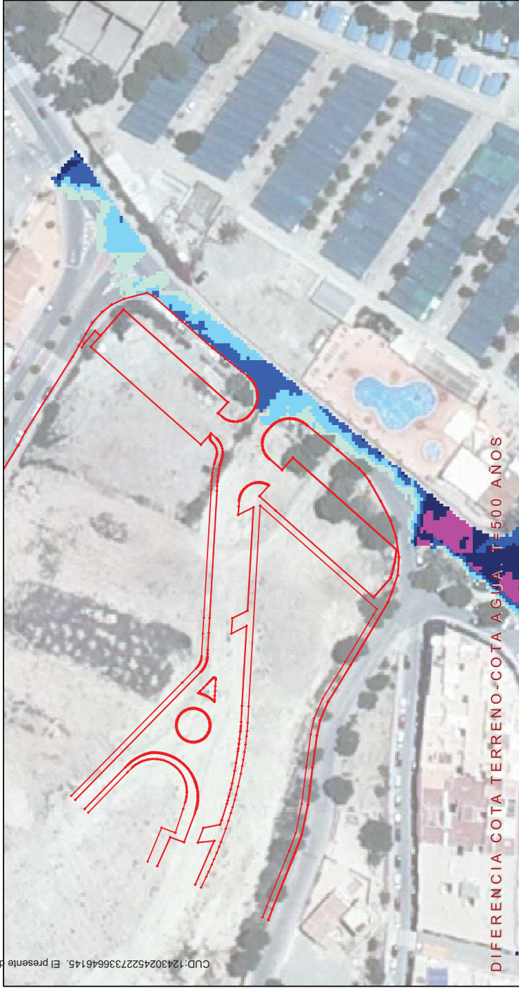
COTAS DEL AGUA. T=500 AÑOS. SNCZI
